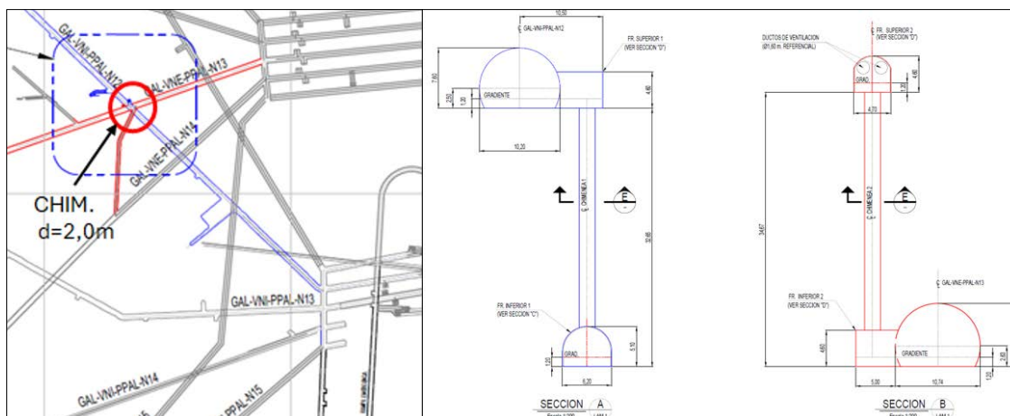
Figura 3: Chimeneas de ventilación diámetro 2 m.
