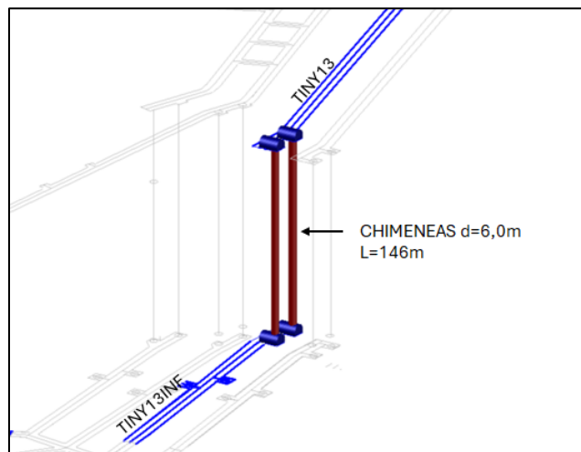
Figura 2: Chimeneas de ventilación del Contrato
