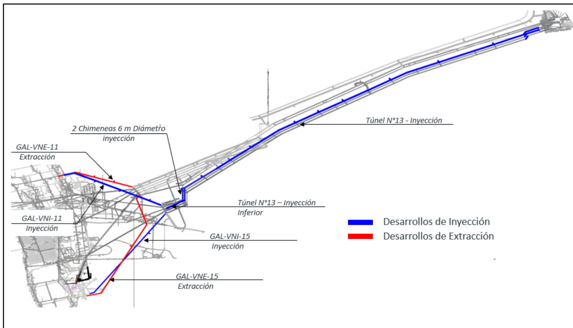
Figura 1: Alcance del Contrato
